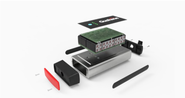
电动自行车电池组 应用于: 电动自行车、电动助力车 电 芯 品 牌: Panasonic/Samsung/Maxell/LG/国产定制电芯 电 芯 类 型: 18650 电 压: 12V/24V/36V/48V 容 量: 6Ah~40Ah 尺 寸: 根据产品定制 充 电 温 度: 0~45 工 作 温 度: -40°C~+60°C 工 作 电 流: 2A~300A 是否含通信: 可按要求实现I2C HDQ SMBUS RS485 RS232 通信 优 势: 配套开发/电流可选/通信/高精度芯片/精确数据传输/温度控制
